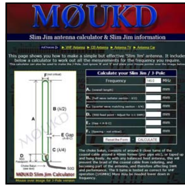
Arriba: Página web del M0UKD calculadora, y la imagen de la antena Slim Jim autoconstruida. Abajo: Esquema y medidas de la Slim Jim y el esquema de una J-Pole sin medidas
